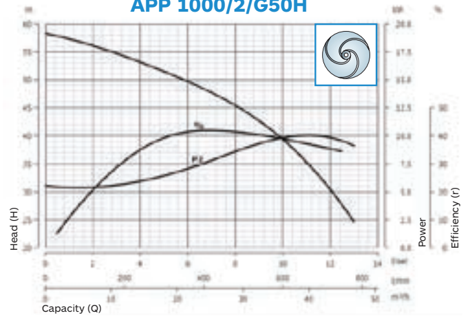
APP 1000/2/G50H
