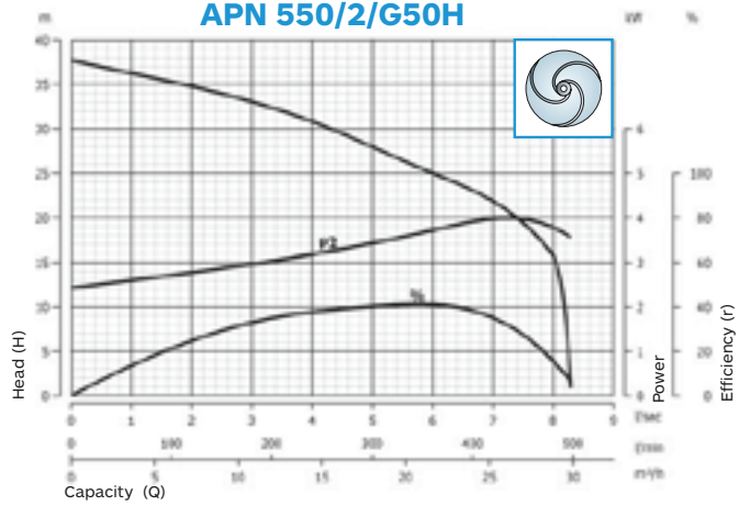
APN 550/2/G50H
