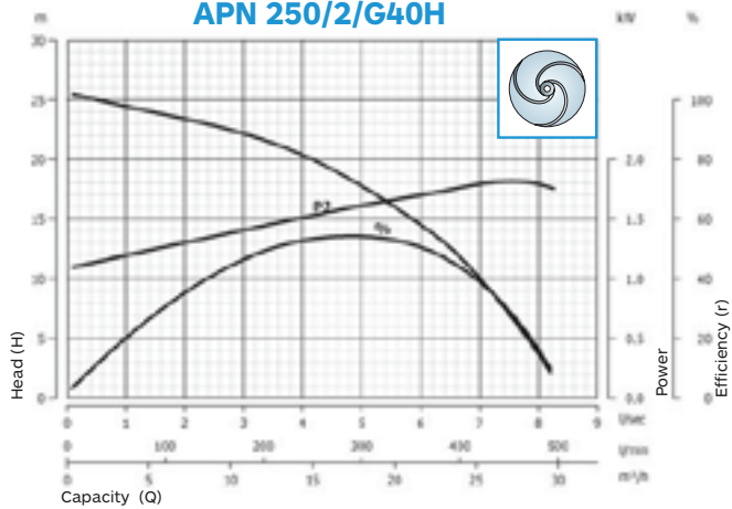
APN 250/2/G40H
