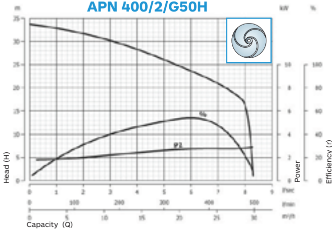
APN 400/2/G50H
